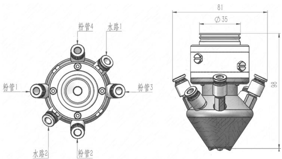
四路送粉喷嘴组件
