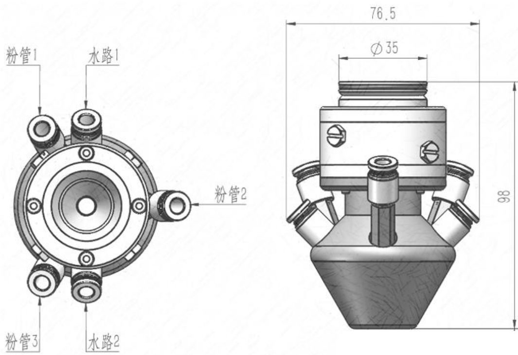
三路送粉喷嘴组件
