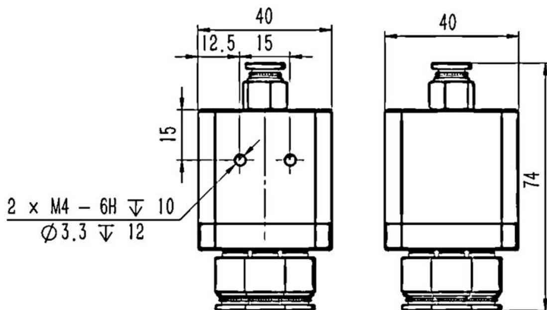
四路送粉器
