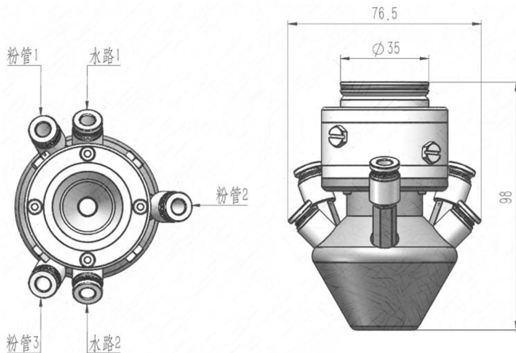
三路送粉喷嘴组件
