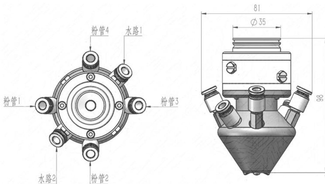
四路送粉喷嘴组件
