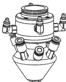
四路送粉喷嘴组件
