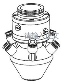
三路送粉喷嘴组件
