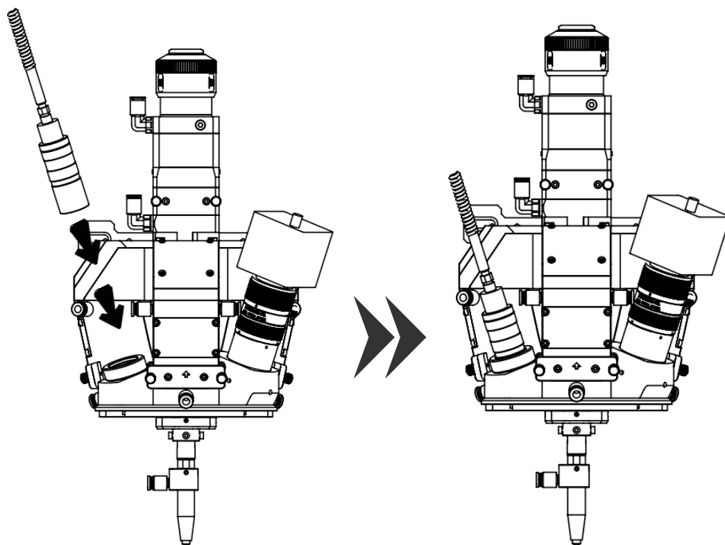
红外测温仪探头安装示意图
