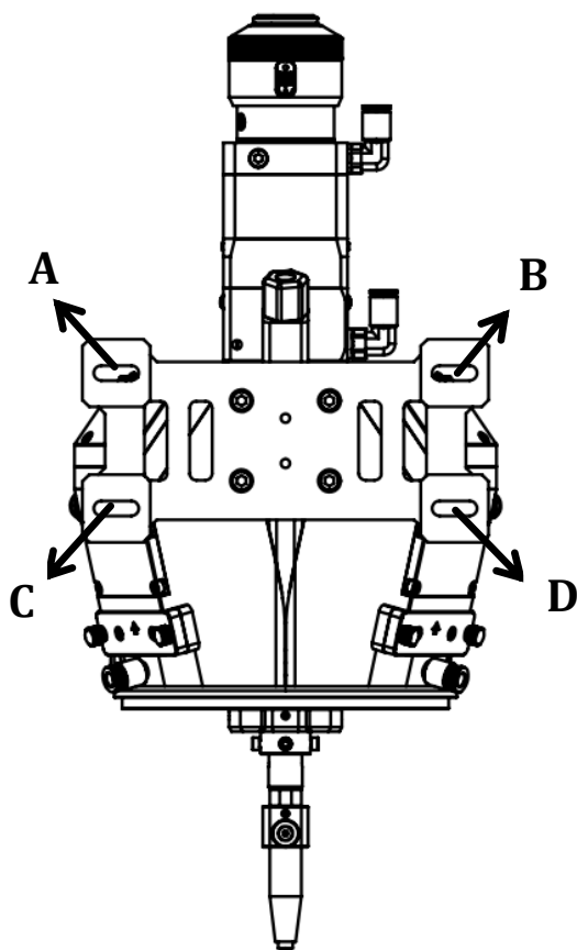
BP06K 激光头反面示意图
