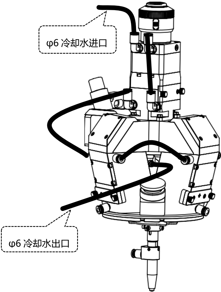
BP06K 激光头冷却水接法
