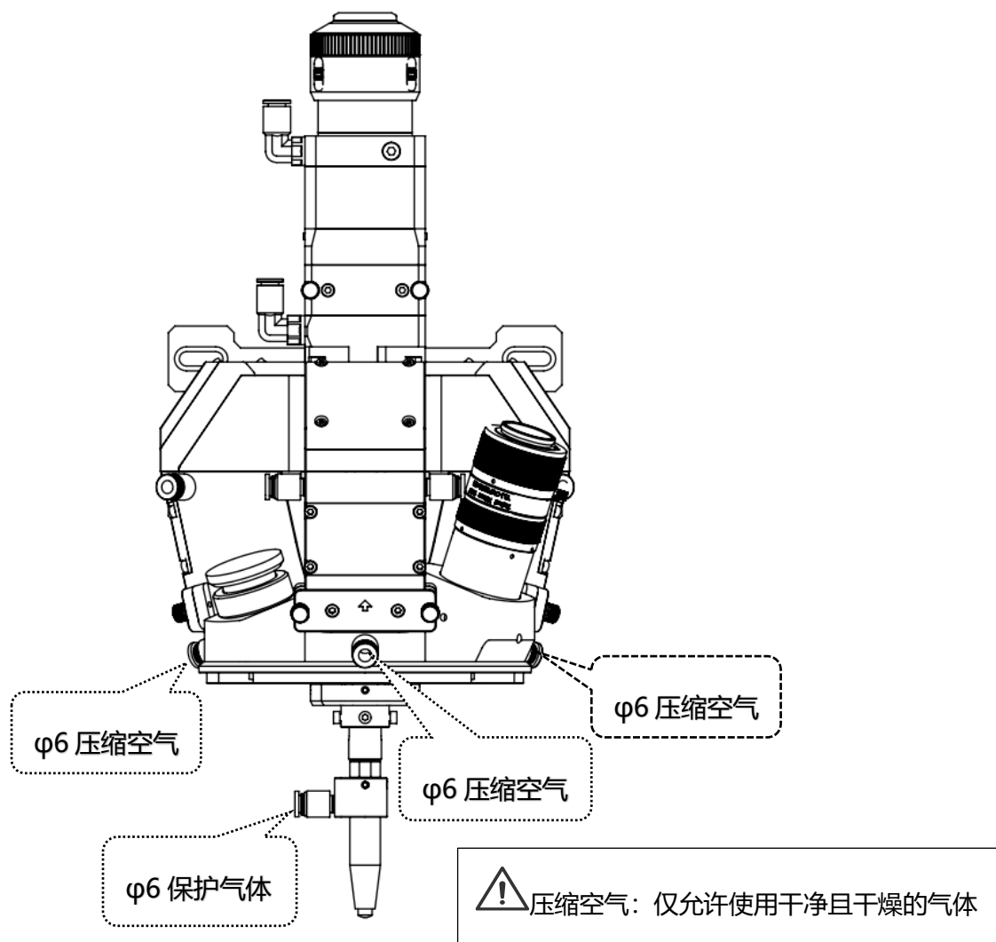
BP06K 激光头气路接法
