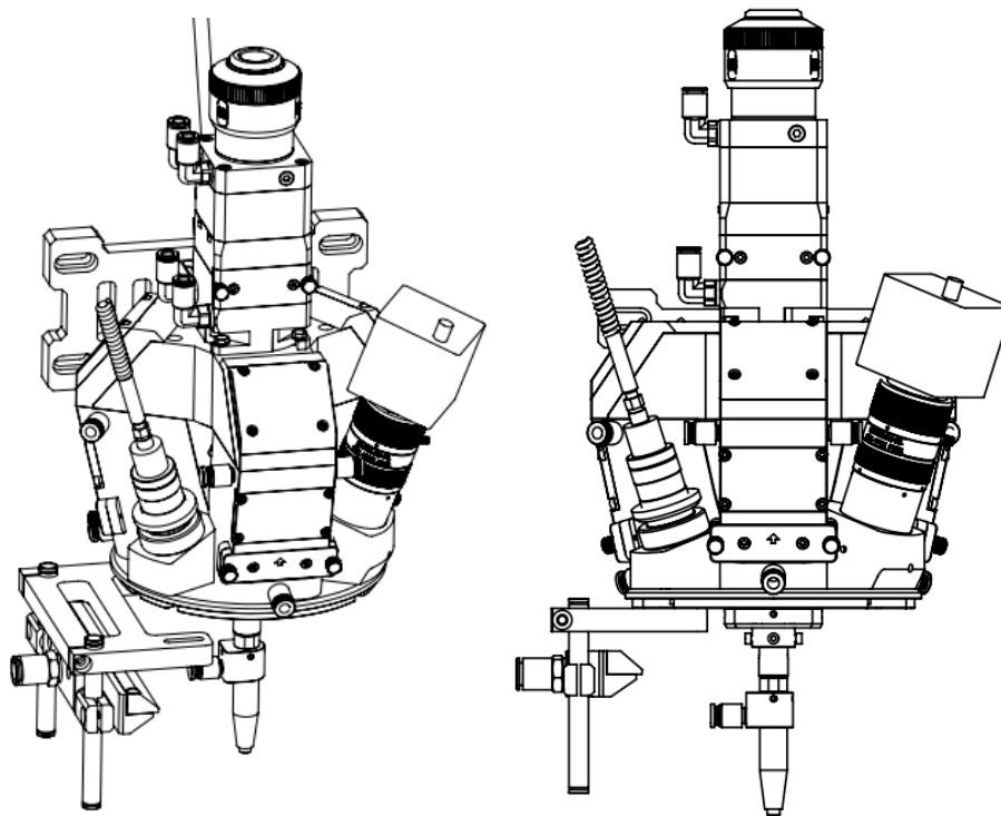
气刀组件安装示意图
