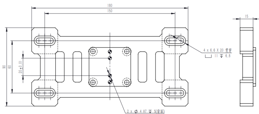
安装背板尺寸图
