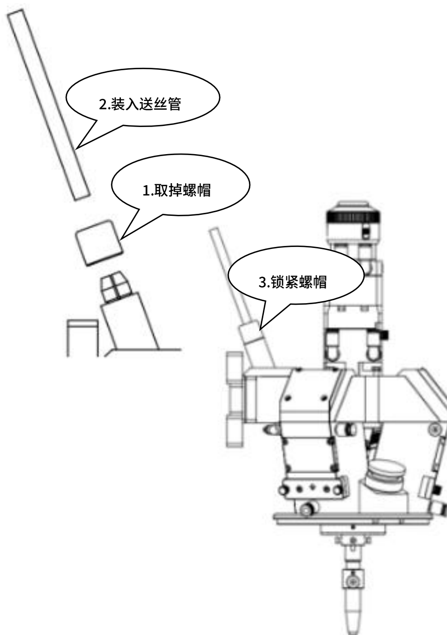
送丝管安装示意图
