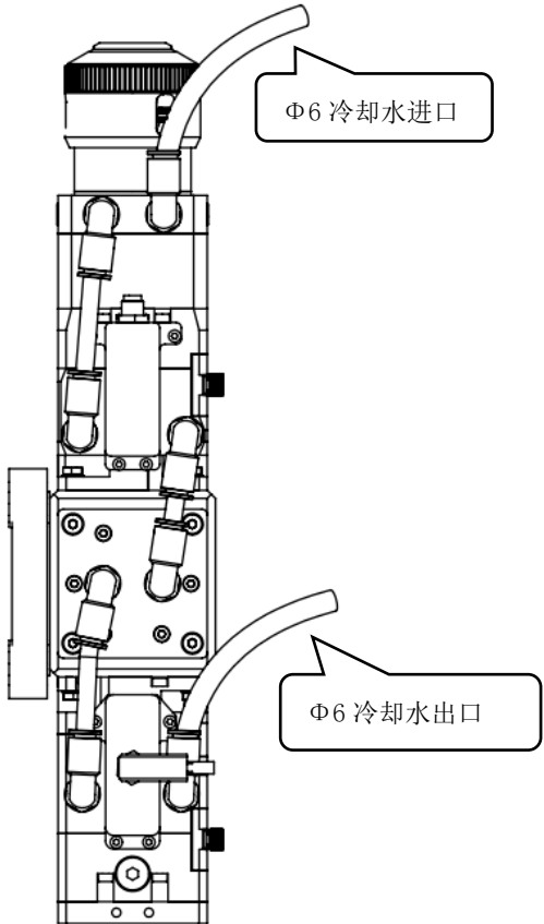
BW06K 激光焊接头冷却水接法
