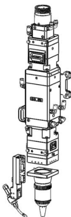
F300 直吹+送丝组件
