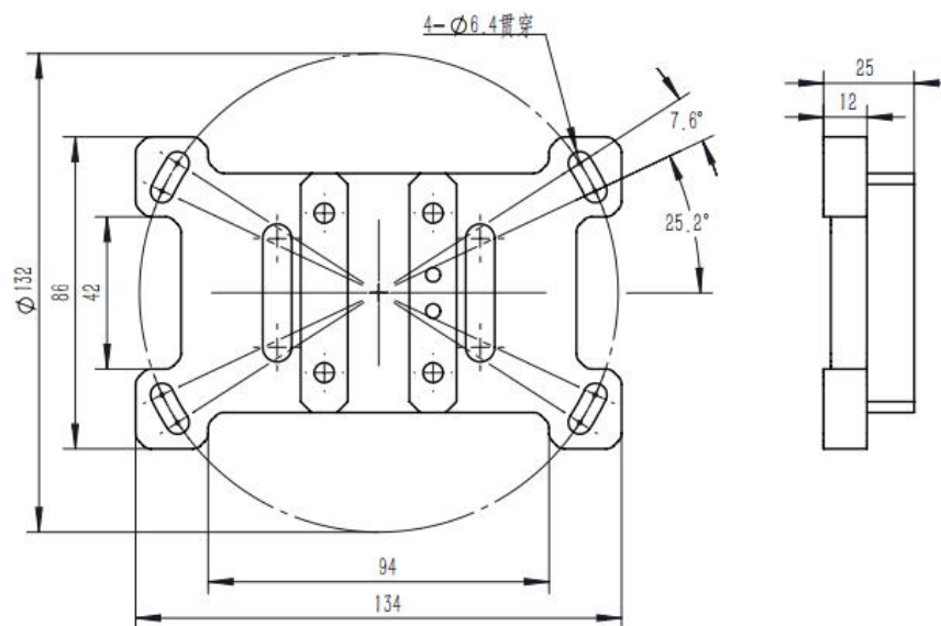
安装背板机械尺寸图
