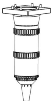
直吹组件
