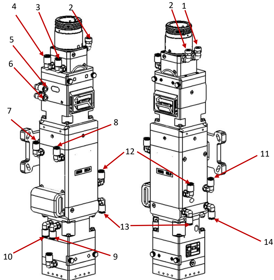
BW06K 四焦点激光焊接头冷却水接法
