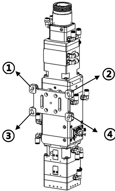
BW06K 四焦点焊接头背面图
