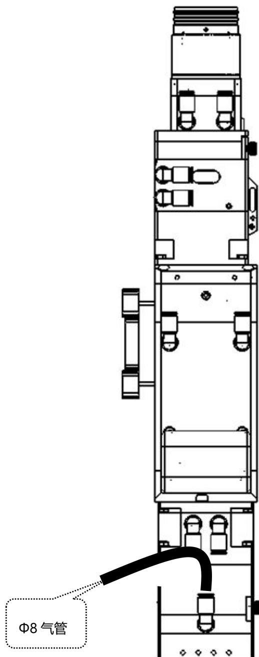
BW06K 四焦点激光焊接头气路接法
